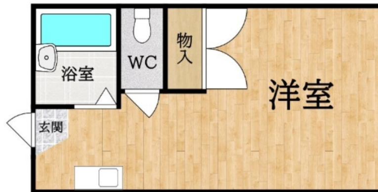
【間取り図】
